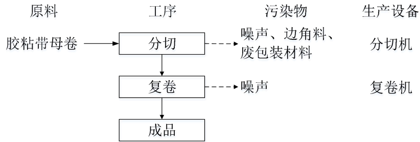
图 2-2 胶粘带生产工艺流程图
