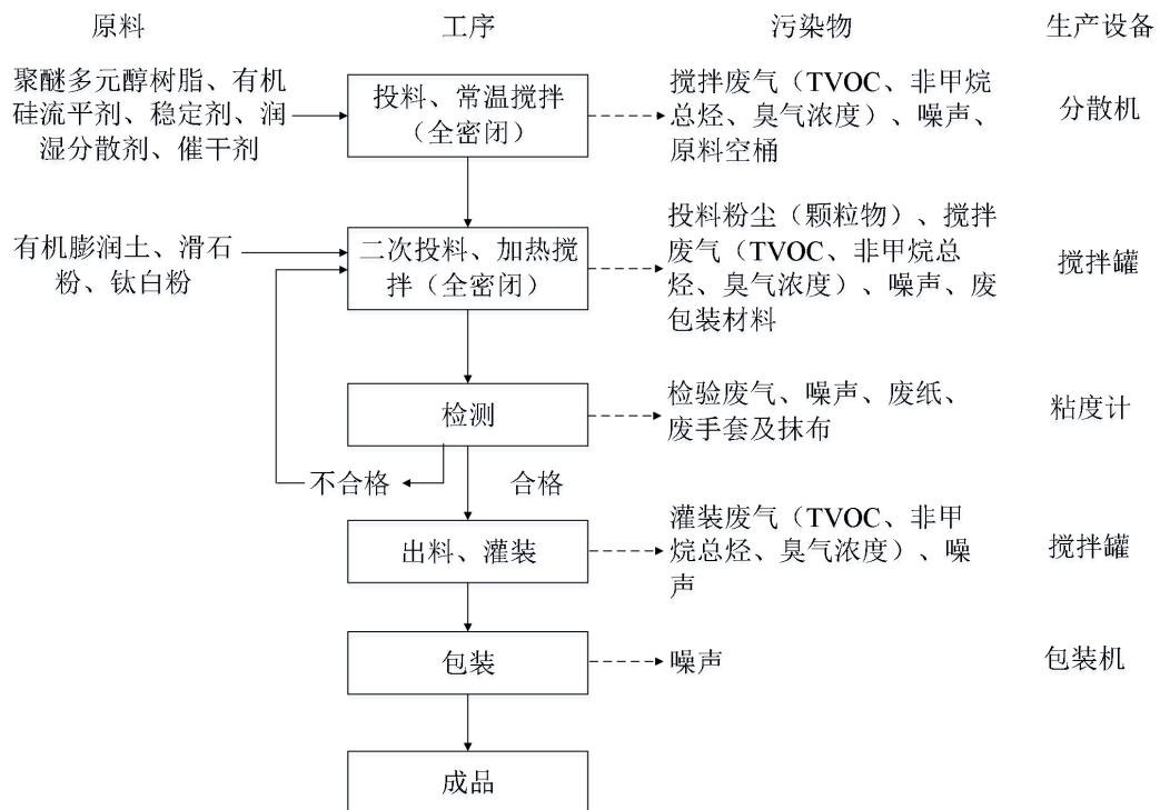
图 2-3 固态灰生产工艺流程图
