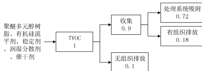
图 2-1 总 VOCs 平衡图（单位：t/a）
