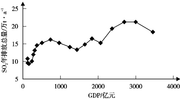
图 1 1985~2002 年广州市 \text{SO}_2 年排放总量与 GDP 的关系
