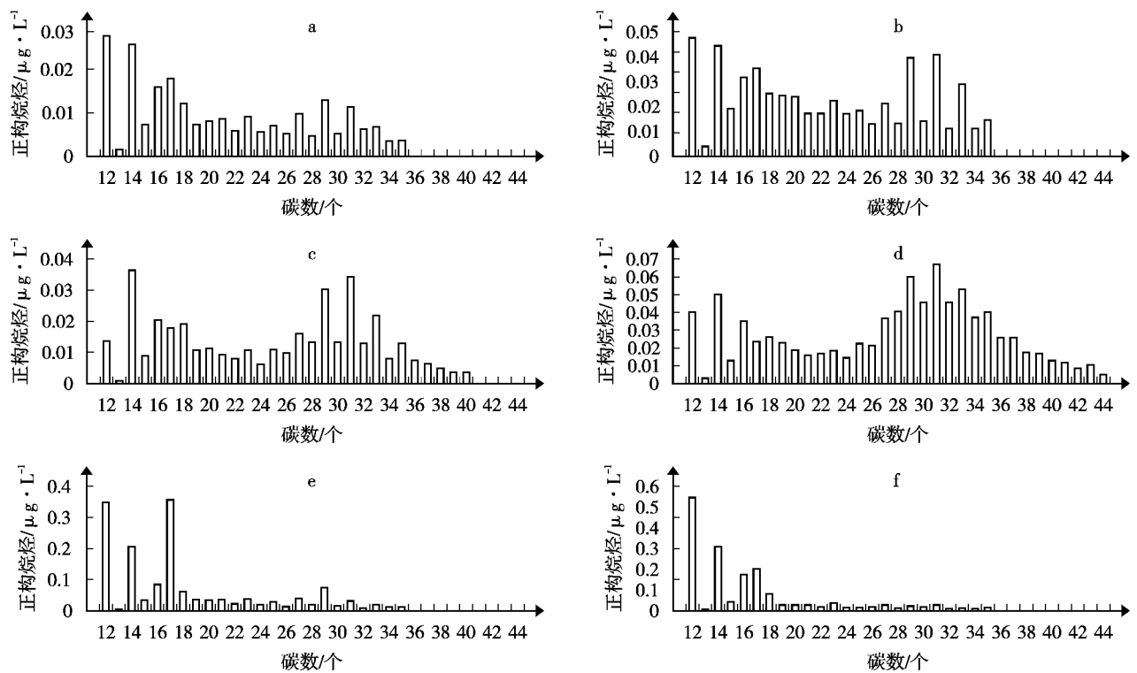
a. A 水厂 b. B 水厂 c. C 水厂 d. D 水厂 e. E 水道 f. F 水道 图 3 某市饮用水水源及河涌水正构烷烃系列化合物分布图
