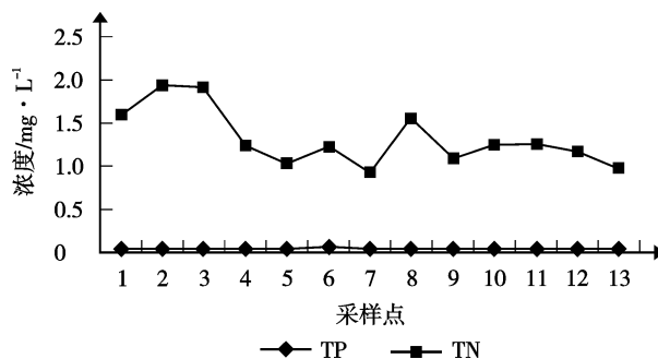
图 2 2002 年总氮、总磷在各采样点的变化
