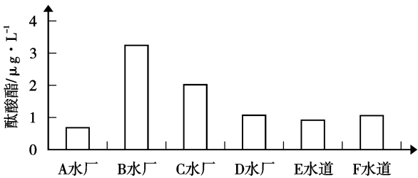
图 2 某市饮用水水源水及河涌中酞酸酯的含量
