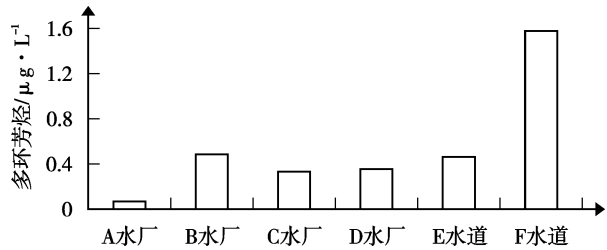
图 1 某市饮用水水源及河涌水中多环芳烃的含量
