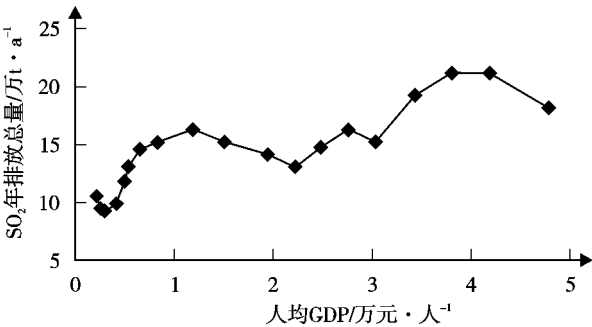
图 2 1985~2002 年广州市 \text{SO}_2 年排放总量与人均 GDP 的关系
